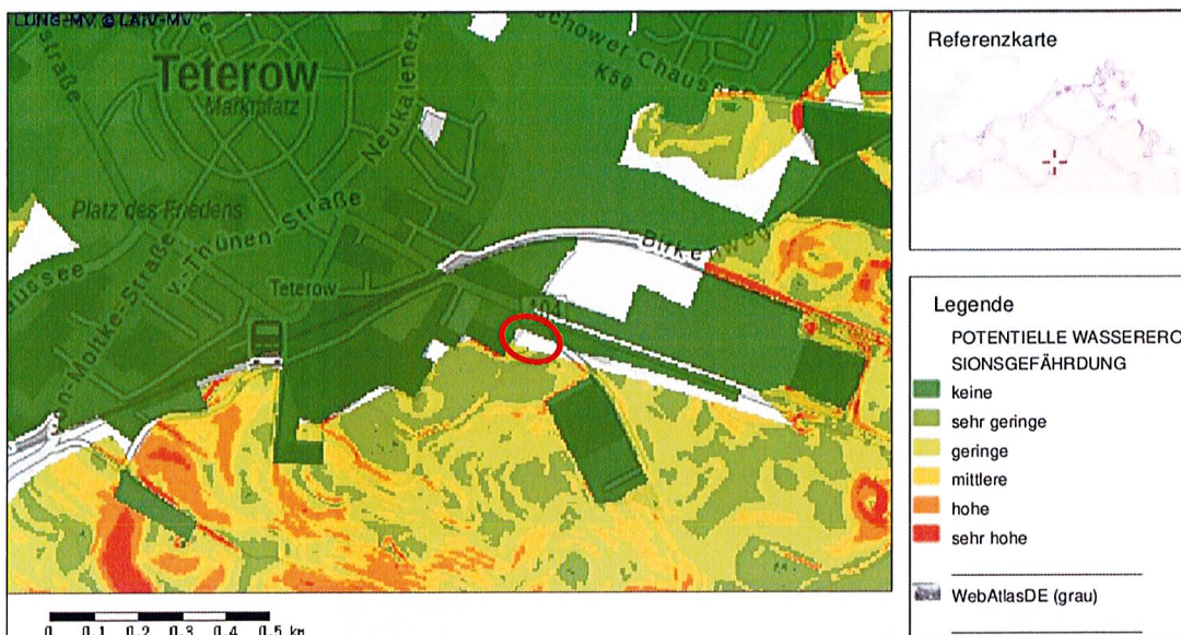
Abb. 7: Wassererosionsgefährdung (Quelle: https://www.umweltkarten.mv-regierung.de/atlas/script/index.php )
