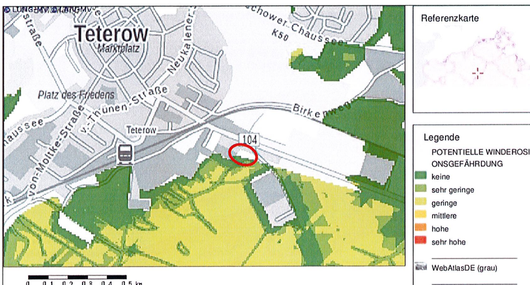
Abb. 8: Winderosionsgefährdung (Quelle: https://www.umweltkarten.mv-regierung.de/atlas/script/index.php )
